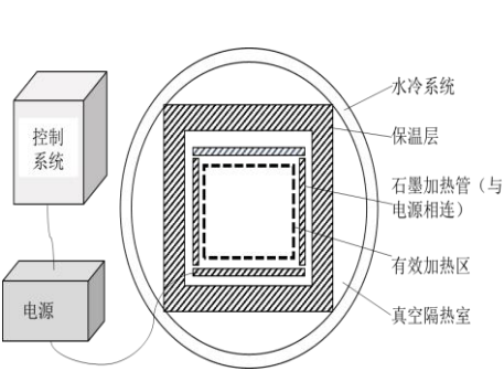
图 1：结构示意图
