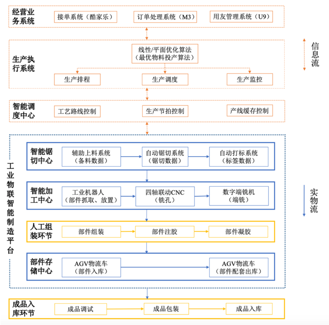
公司智能制造系统业务流程图
