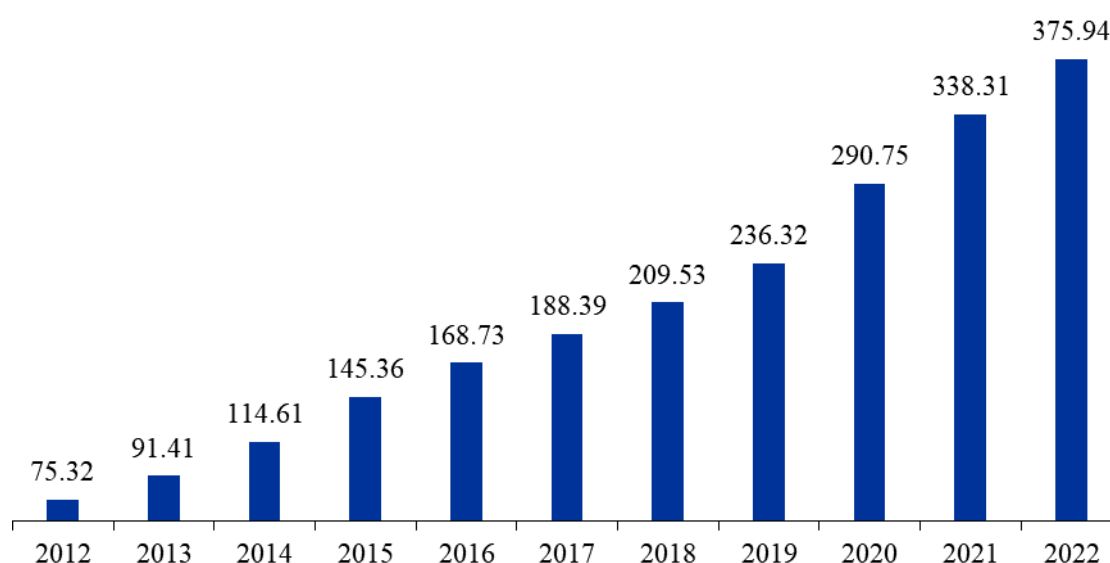
2012-2022 年底我国累计风电装机容量（GW）
