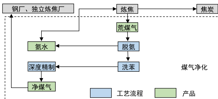
图：煤气净化工艺流程
