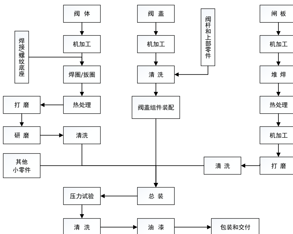
(3) 闸阀工艺流程图
