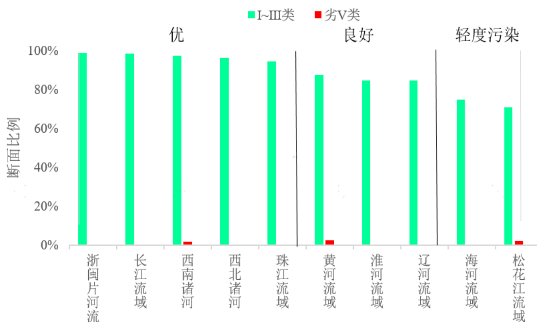
2022 年 1-12 月七大流域和西南、西北诸河及浙闽片河流水质类别比例
