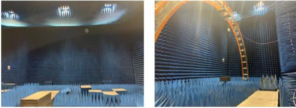
电磁参数测试平台
