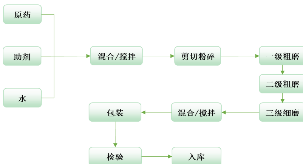
(4) 悬浮剂生产工艺流程图
