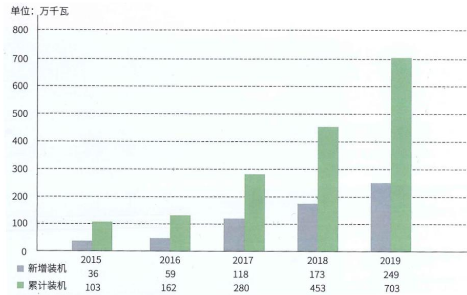
图：我国海上风电新增及累计装机容量
