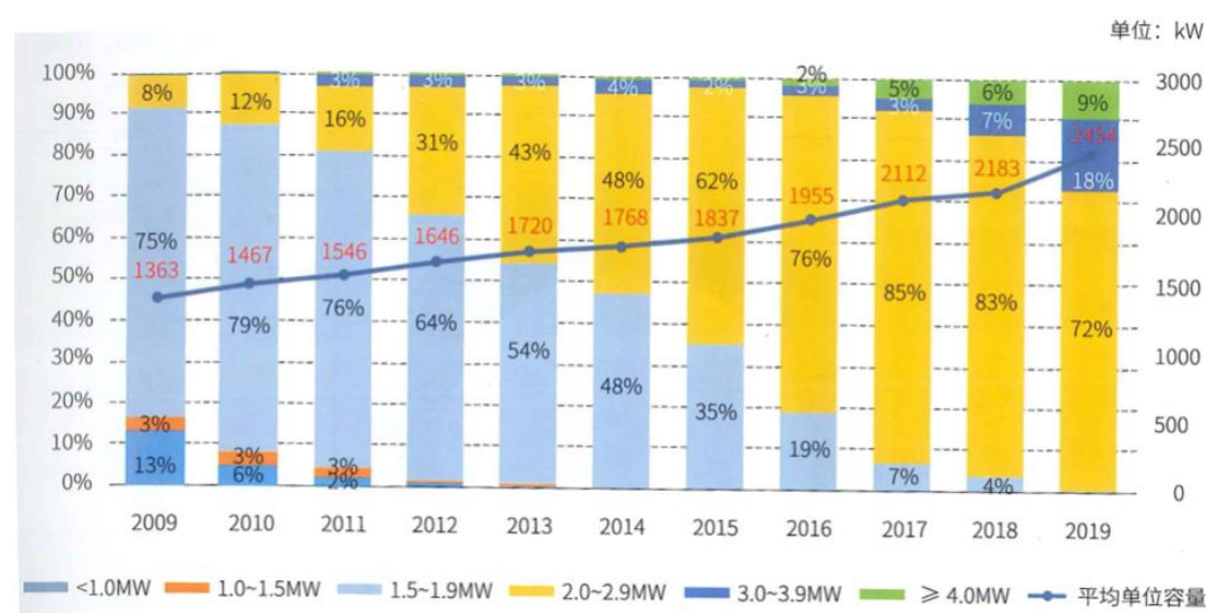
图：我国 2009-2019 年新增风机容量结构变化
