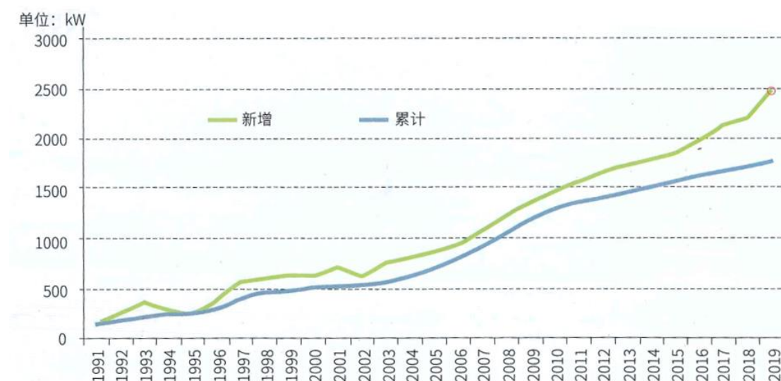
图：我国 1991-2019 年全国新增和累计装机风电机组平均单机容量变化
