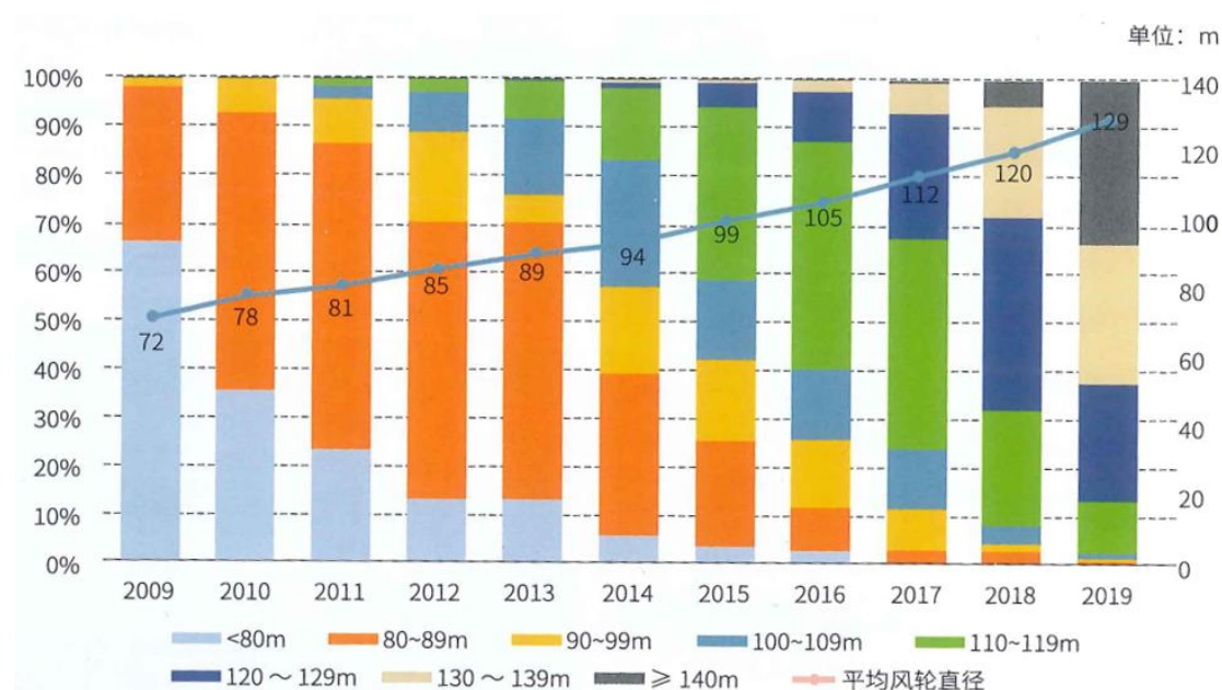
图：2009-2019 年全国新增风电机组不同风轮直径装机容量占比变化
