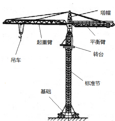
塔式起重机
