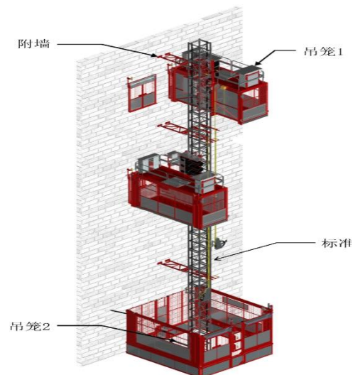
施工升降机
