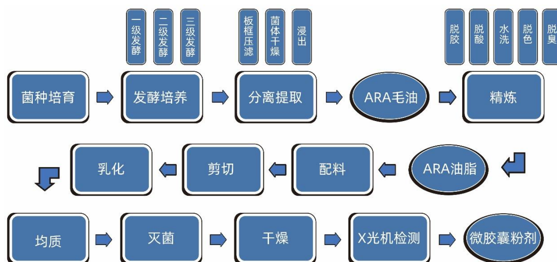
图 6-3：ARA 产品生产工艺流程图
