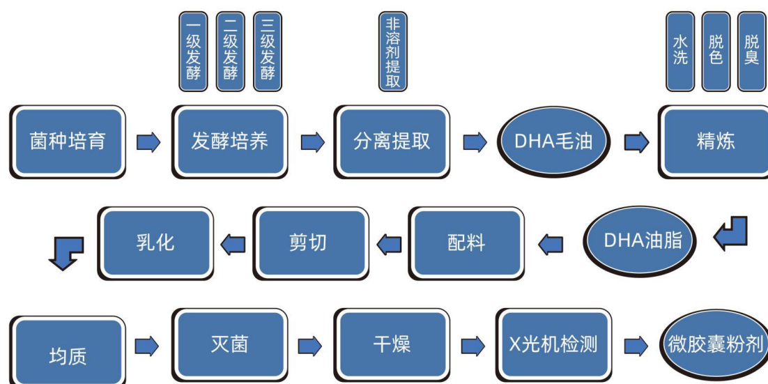
图 6-2：微藻 DHA 产品生产工艺流程图
