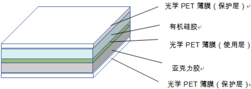
(2) 防蓝光光学功能膜产品结构图
