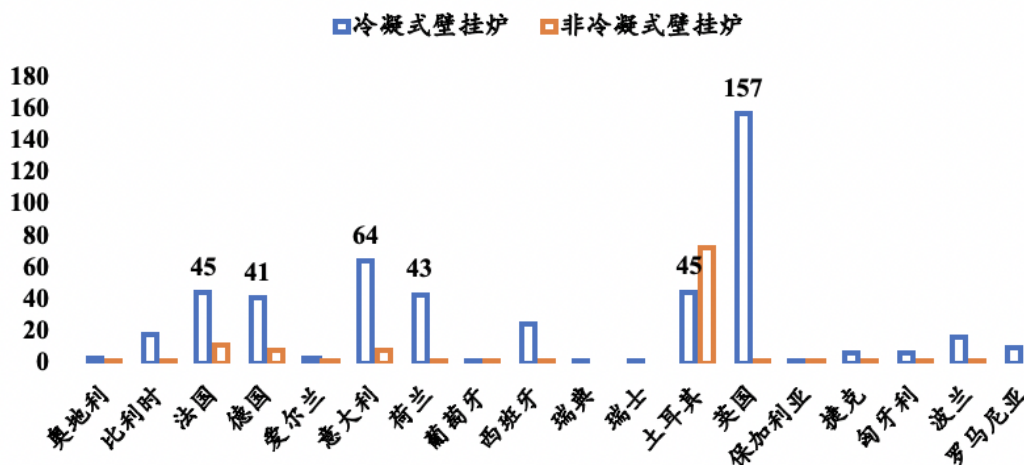
2017年欧洲各国或地区壁挂炉销量（万台）
