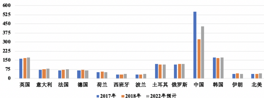
2017~2022年全球燃气壁挂炉市场趋势分析（万台）
