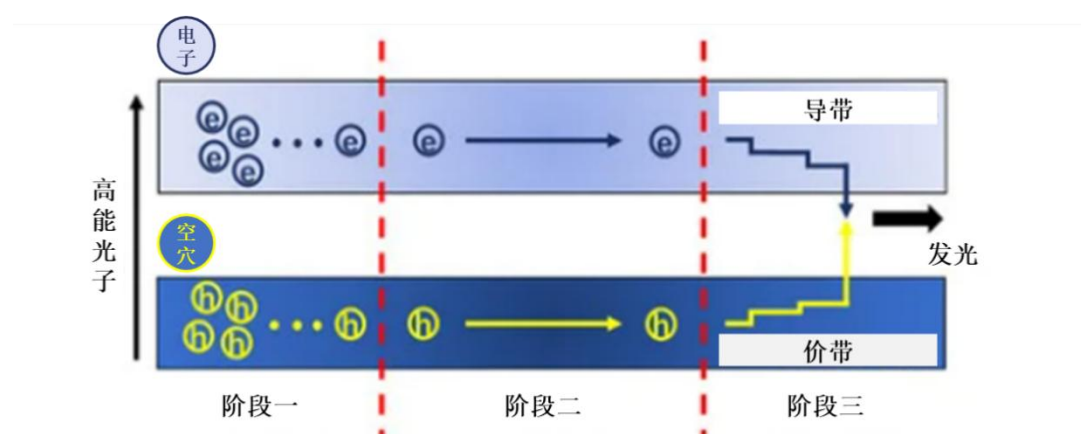
图：闪烁晶体发光原理图
