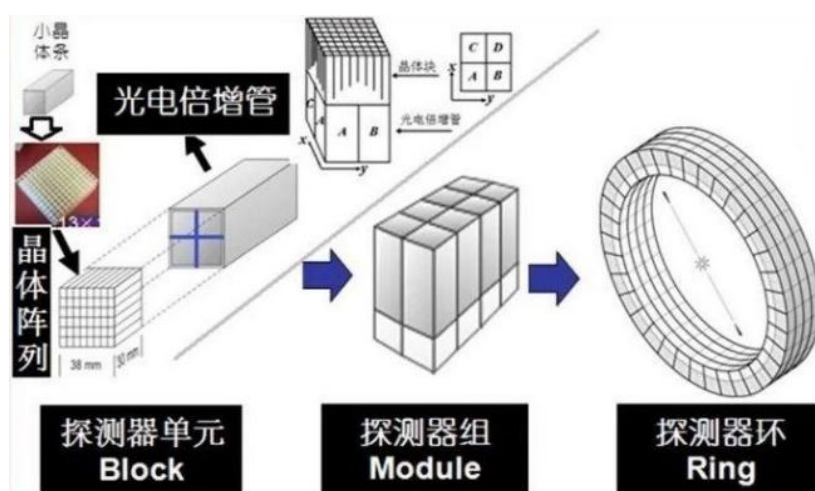
图：硅酸钪镧闪烁晶体工作示意图
