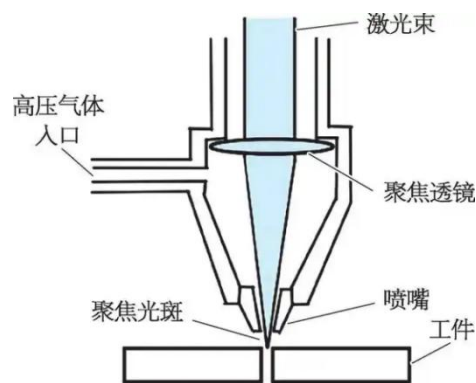
图：激光切割的工作原理
