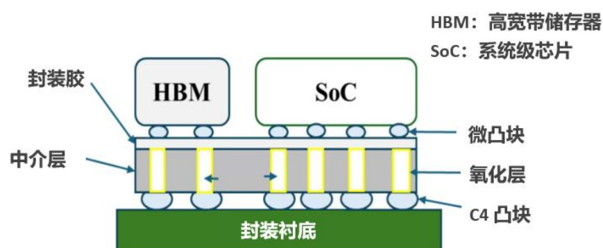
图：CoWoS 先进封装示意图
