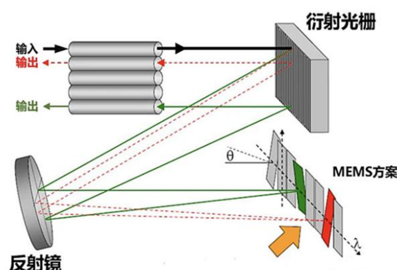
图：MEMS 交换机原理图
