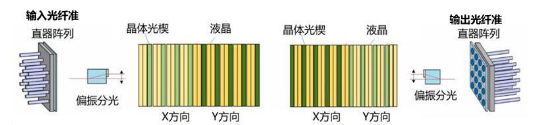
图：数字液晶技术交换机原理图
