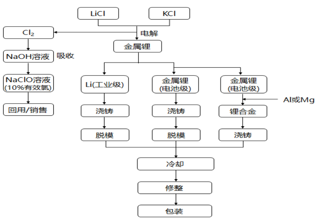
(3) 金属锂生产工艺流程图
