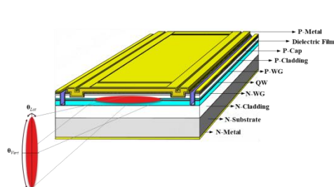
边发射半导体激光芯片
