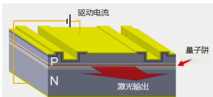
边发射半导体激光芯片工作示意图
