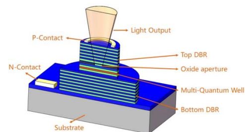
面发射半导体激光芯片
