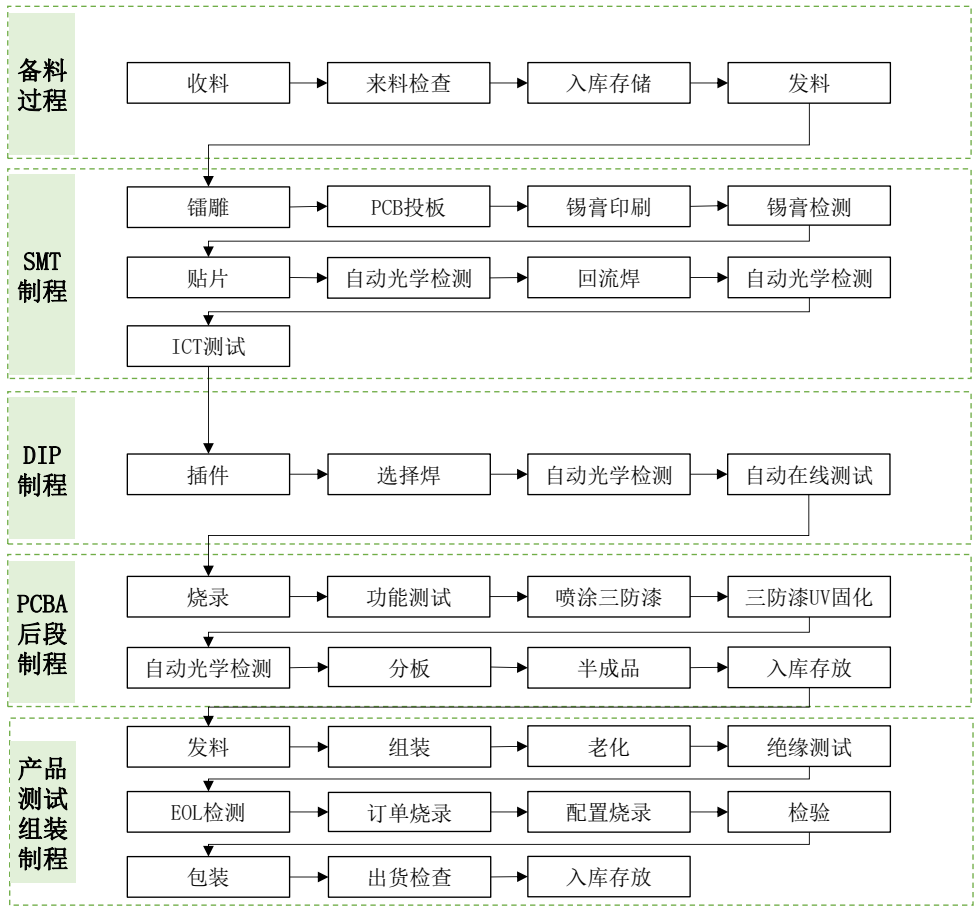
公司主要生产产品的生产工艺流程示意图
