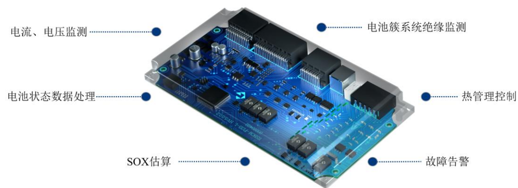
公司电池簇控制管理模块的内部结构及主要功能模块示例图如下：
