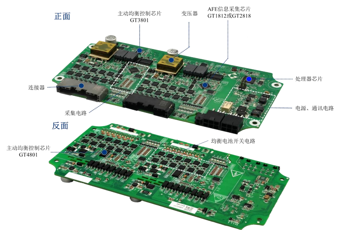
公司主动均衡从控模块的内部结构及主要功能模块示例图如下：
