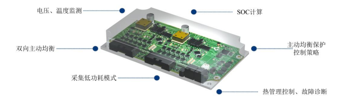
公司主动均衡从控模块的内部结构及主要功能模块示例图如下：
