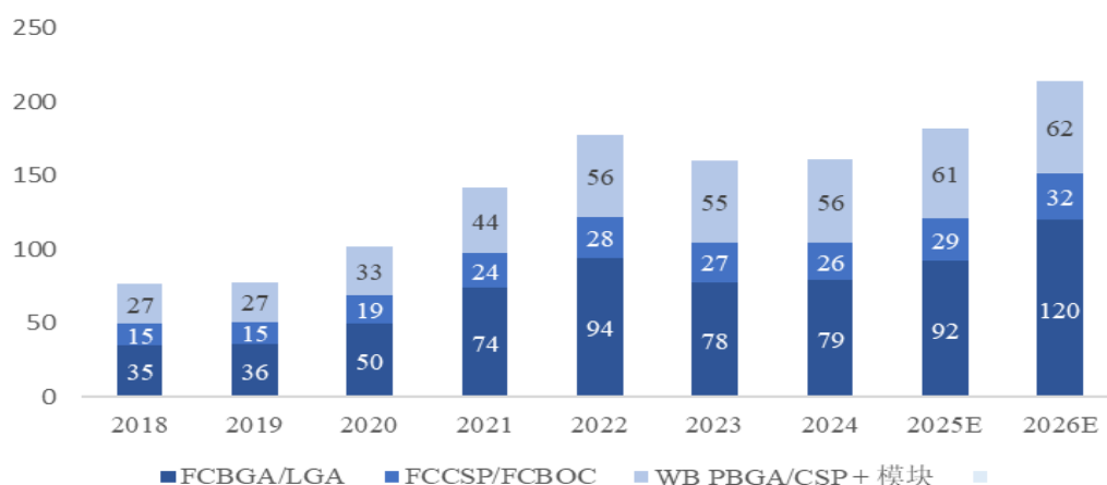
IC封装载板分产品市场规模预测（亿美元）
