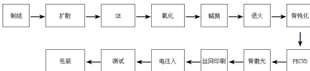
光伏电池片制作流程
