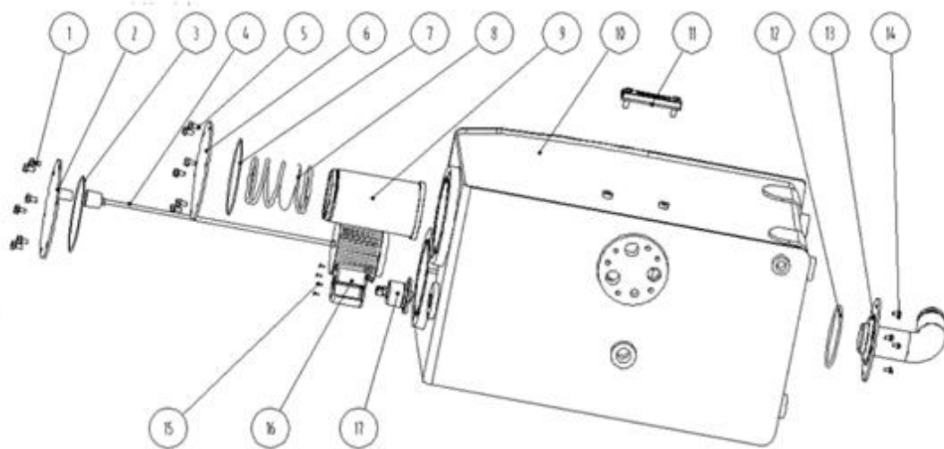
注：1、组合螺栓；2、法兰压盖；3、O型圈；4、吸油过滤器；5、组合螺栓；6、法兰盖；7、O型圈；8、弹簧；9、回油筒、回油过滤器；10、液压油箱箱体；11、液位计；12、O型圈；13、吸油泵管；14、组合螺栓；15、螺钉；16、呼吸阀保护罩；17、呼吸阀
