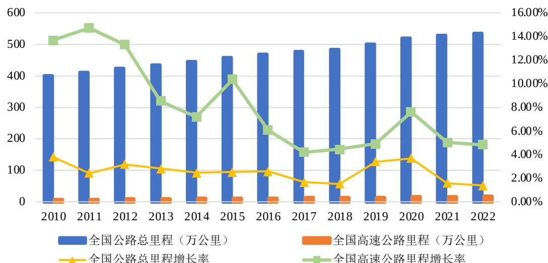
2010-2022年全国公路总里程及高速公路增长情况
