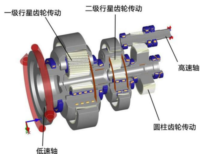
多级行星齿轮传动结构图
