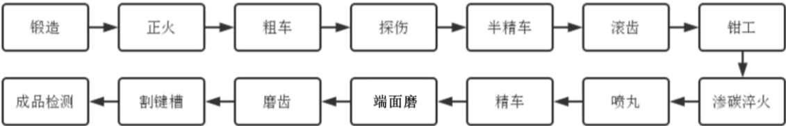
齿轮件产品的工艺流程图
