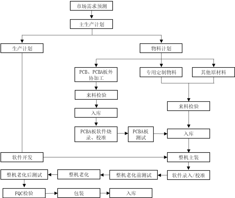
(1) 伺服驱动器和小型 PLC 生产工艺流程图
