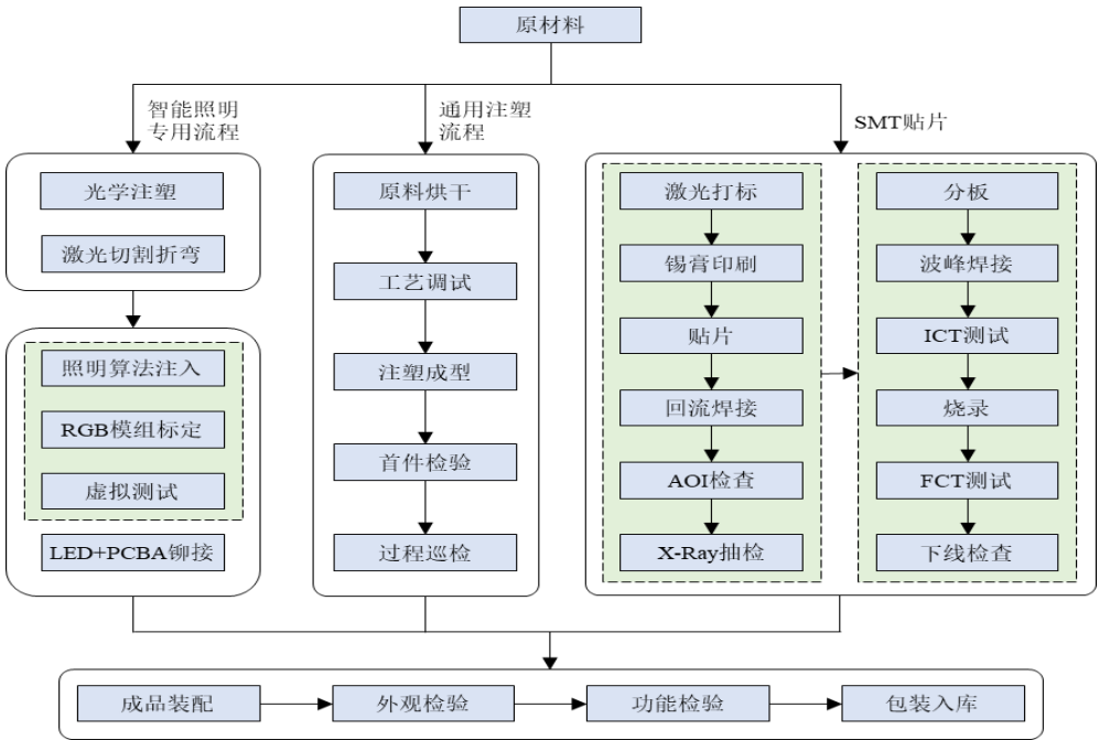
（1）智能光电产品工艺流程图
