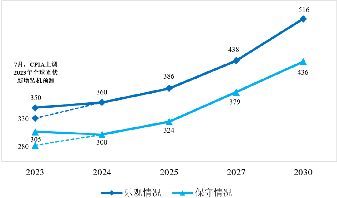
2023-2030 年全球光伏新增装机预测（单位：GW）
