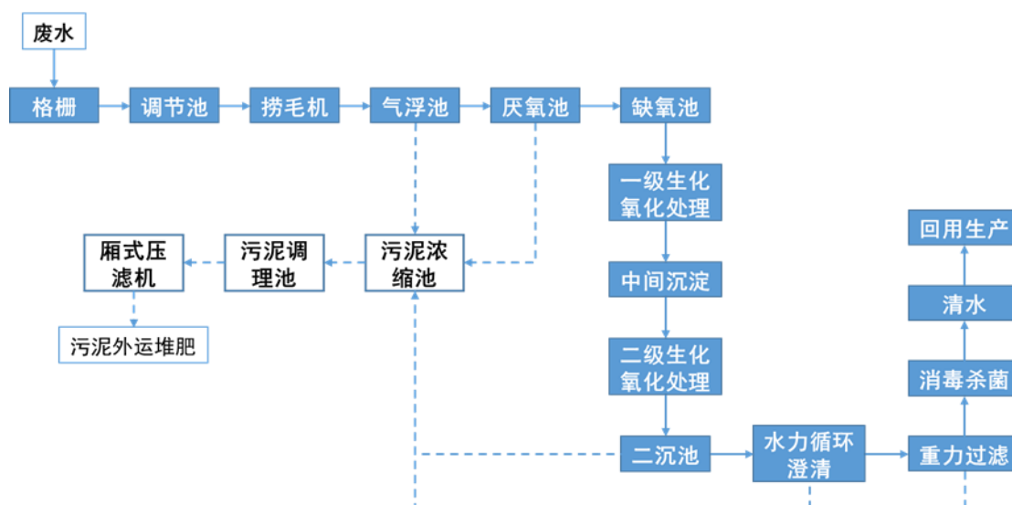
中水回用工艺流程示意图
