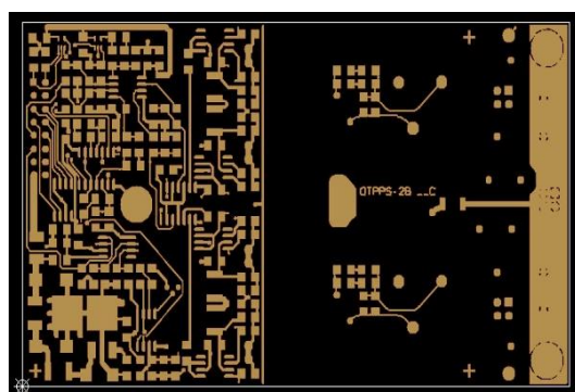
某款厚铜板：
