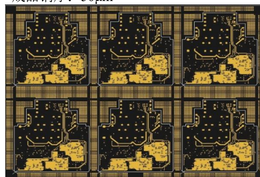
某款 4 层板：
