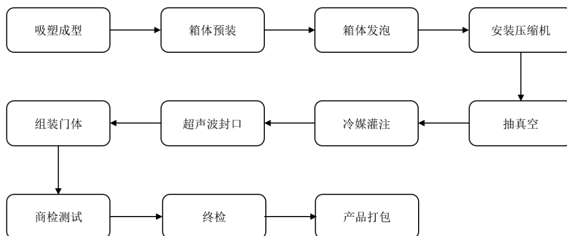
商用展示柜产品工艺流程
