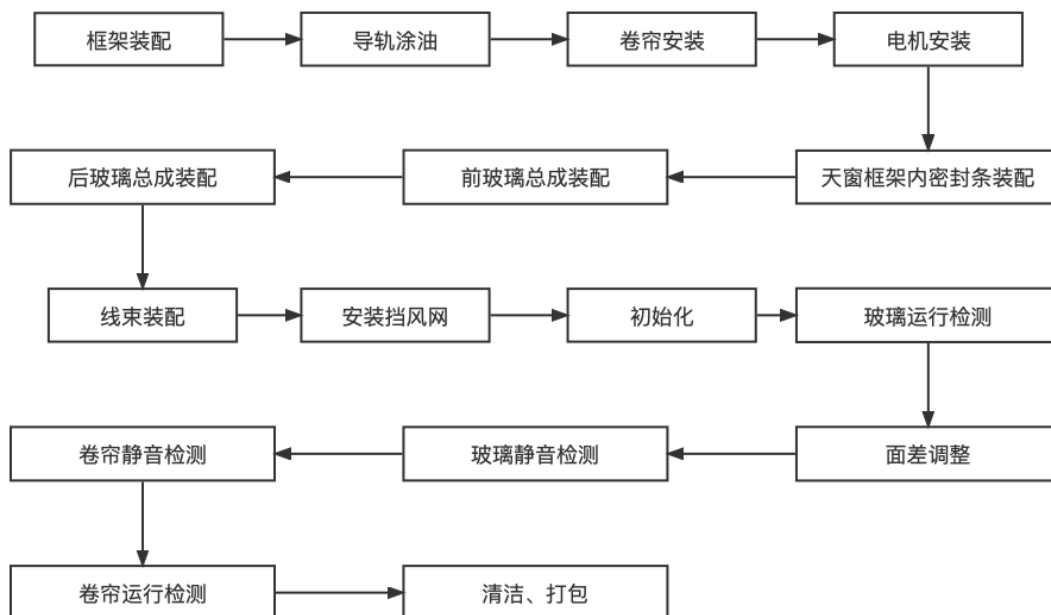
图 5-2 全景天窗总成装配流程图
