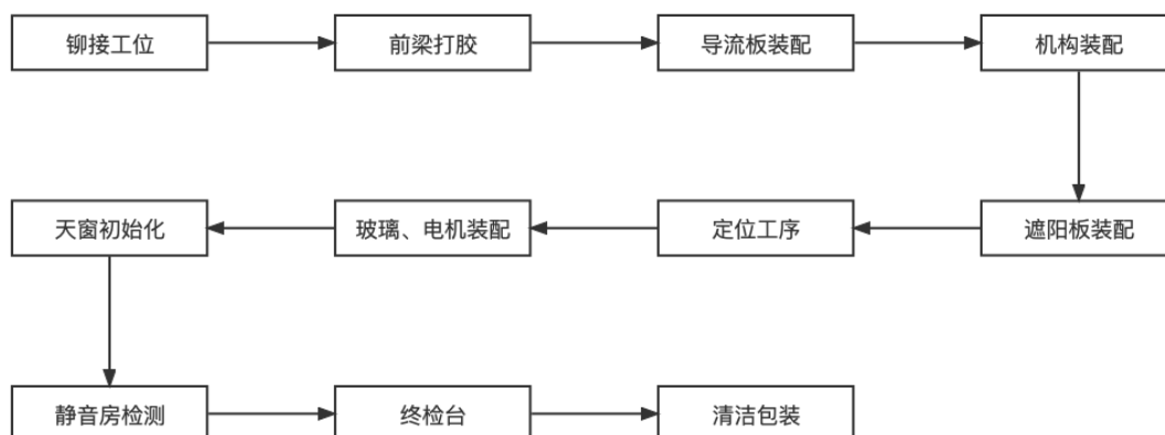
图 5-3 小天窗总成装配流程图
