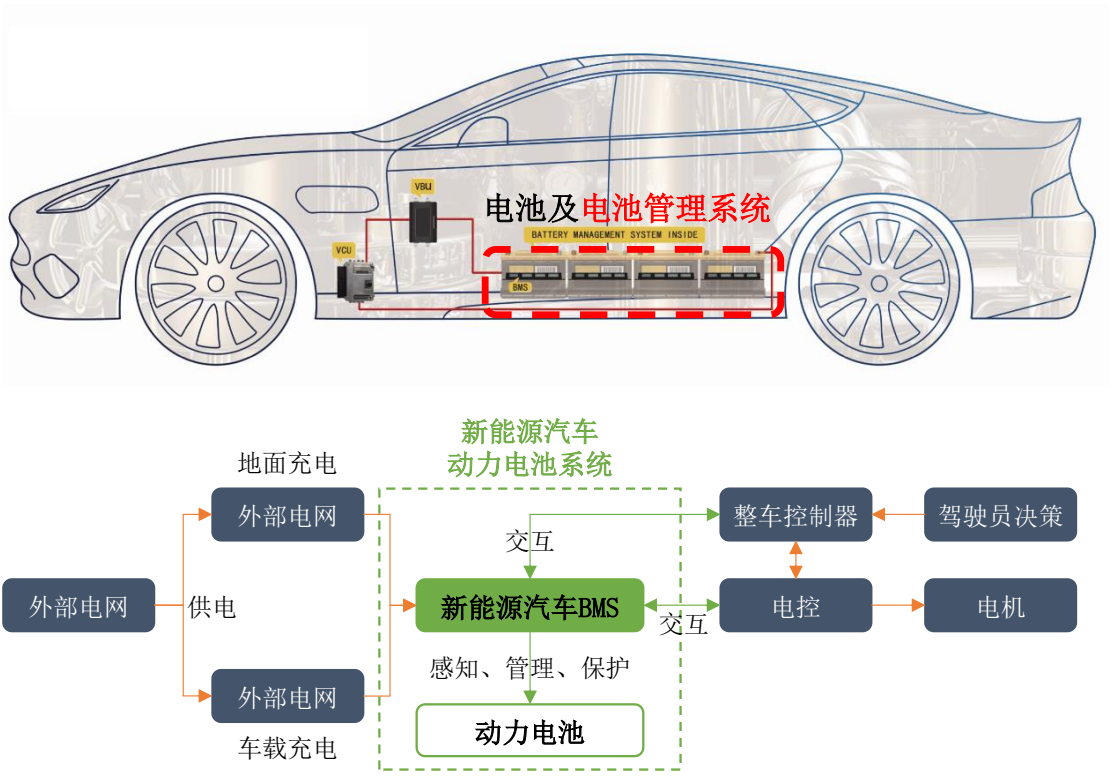
新能源汽车用动力电池 BMS 产品应用示意图
