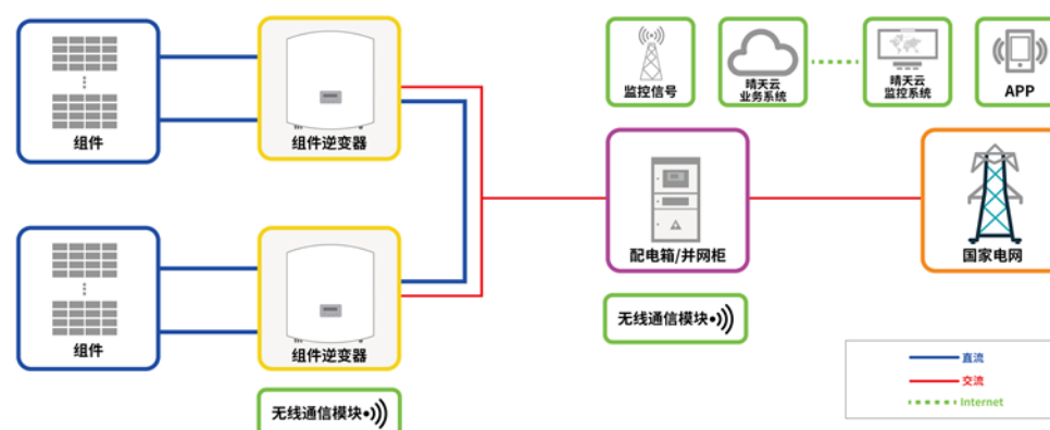
分布式光伏电站接入“晴天云”系统示例
