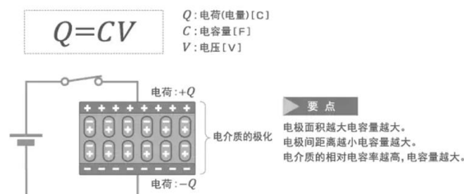
电容器积蓄的电荷
