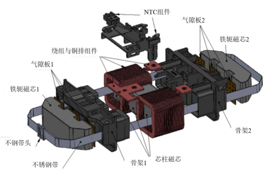
公司车规级升压电感结构示意图
