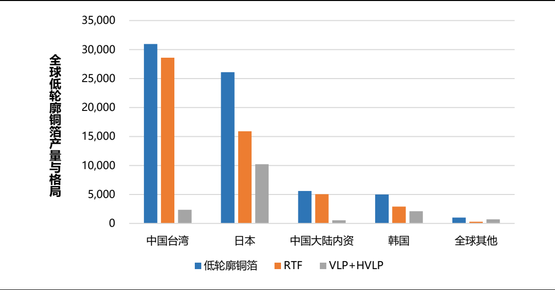
图：2020 年全球低轮廓铜箔产量与格局
