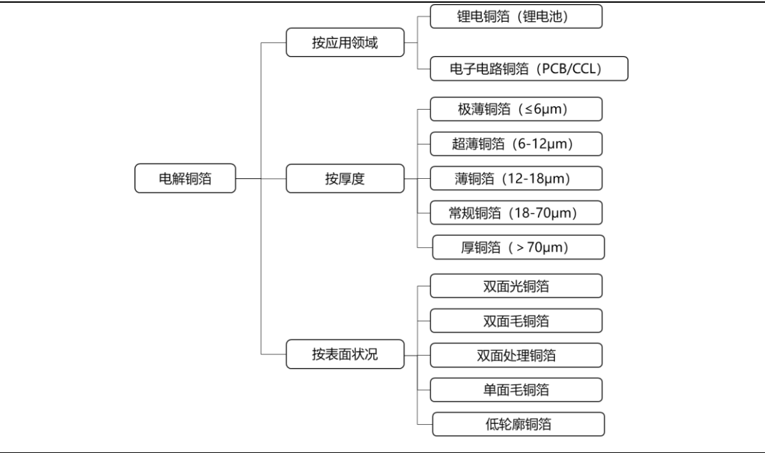
图：电解铜箔分类情况
