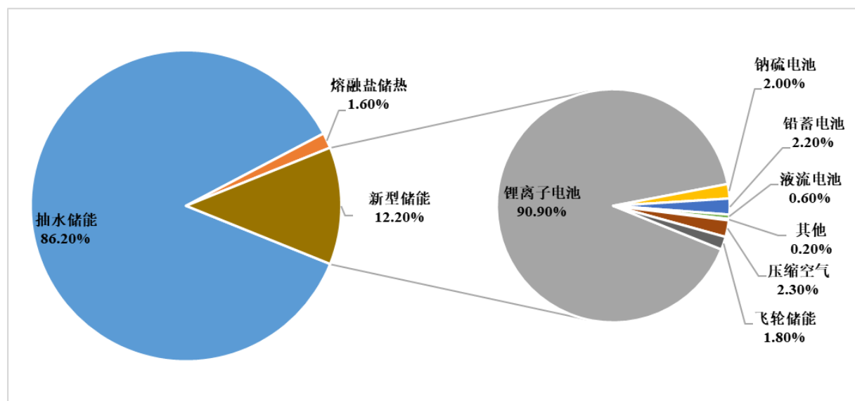
图：2021 年全球储能市场累计装机规模构成；数据来源：CNESA
