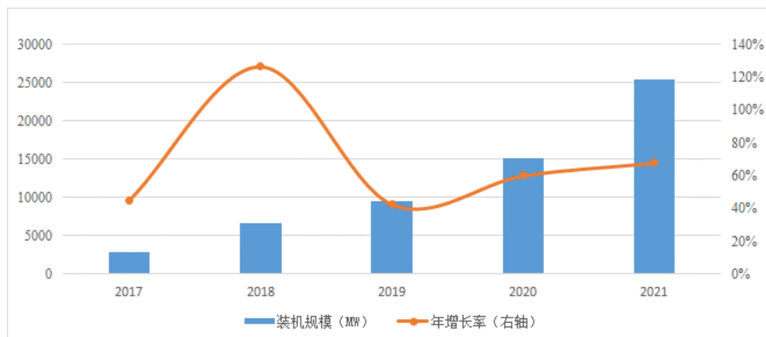
图：2017-2021 年全球新型储能市场累计装机规模（MW，%）；数据来源：CNESA
