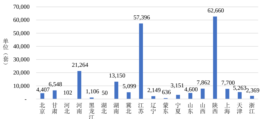
2022年配电终端招标区域分布情况
