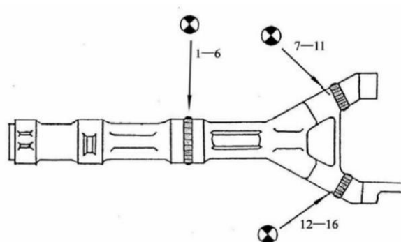
图：主起落架减震支柱外筒焊缝 X 射线检测
