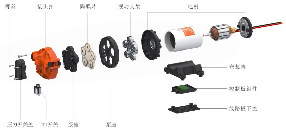
水泵结构图
