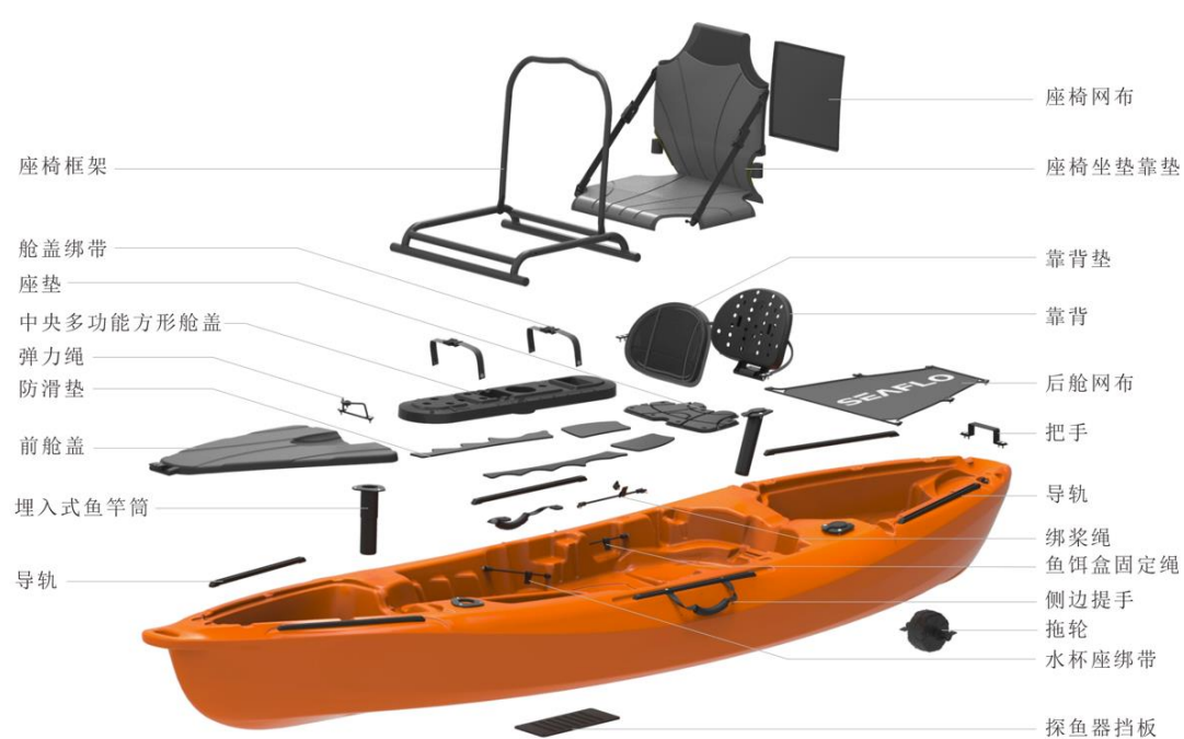
钓鱼艇结构图
