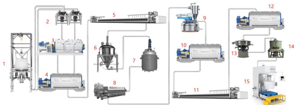
湖南杉杉项目三元材料产线布局如上图，序号与部件的对应关系如下：
