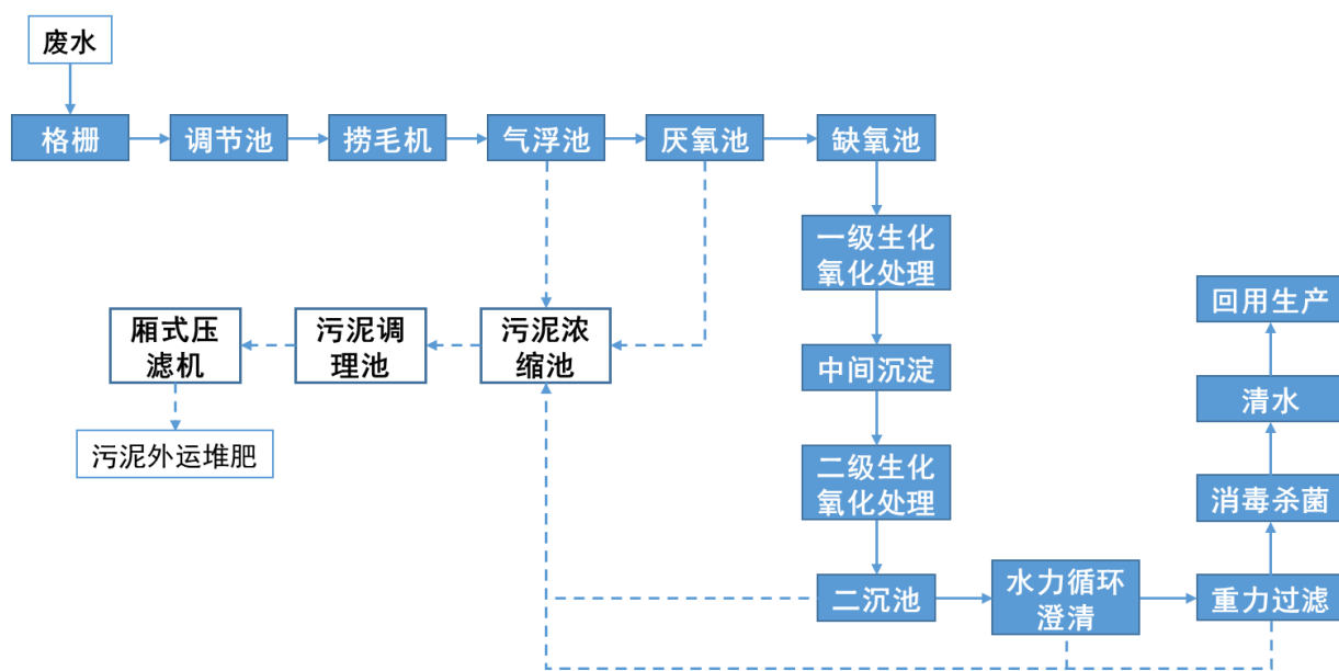
中水回用工艺流程示意图
