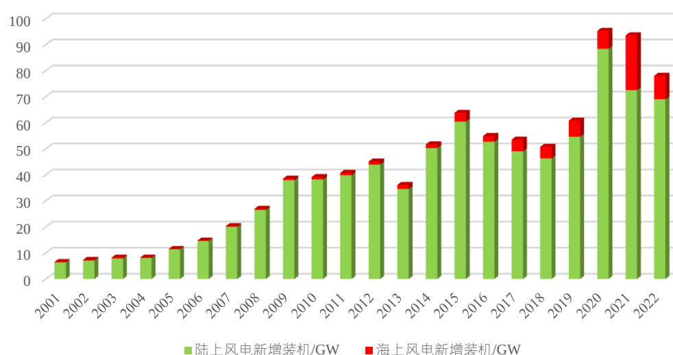
2001年-2022年全球风电新增装机
