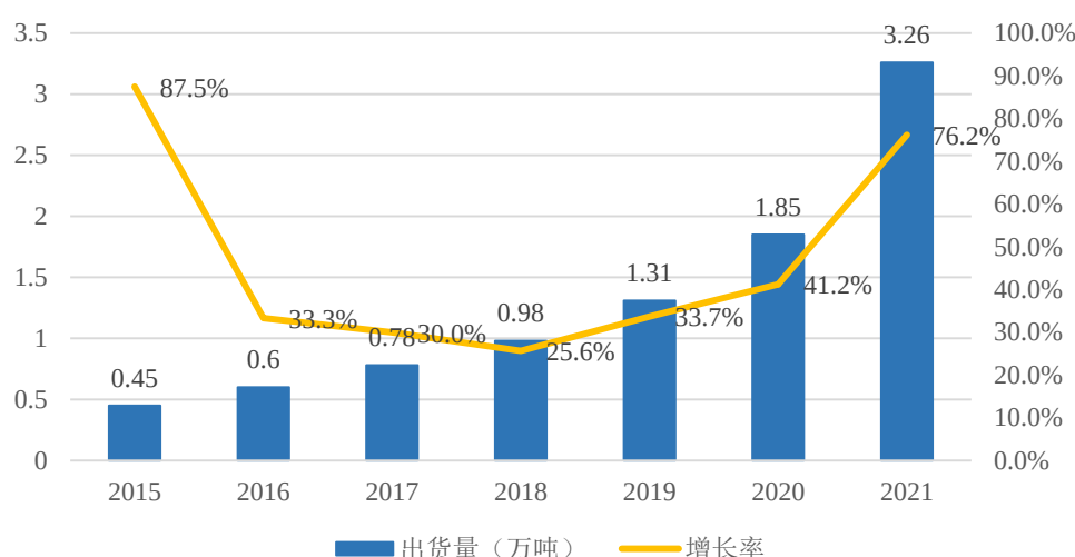
2015-2021 年我国电解液添加剂出货量
