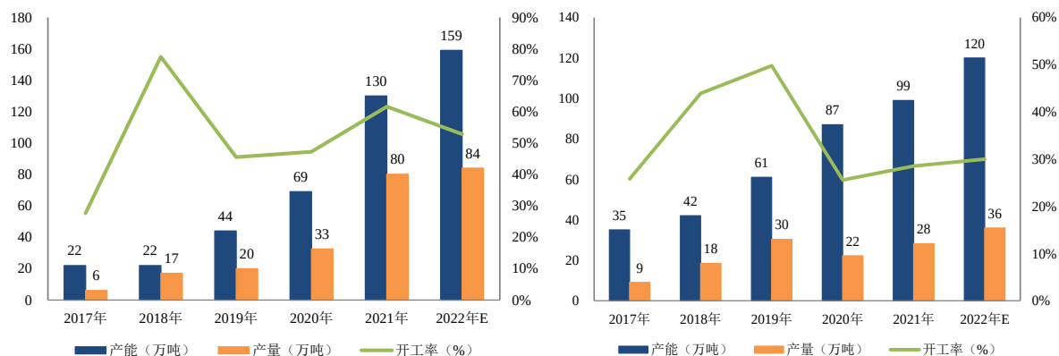
图：中国油系针状焦产能、产量和开工率 图：中国煤系针状焦产能、产量和开工率
