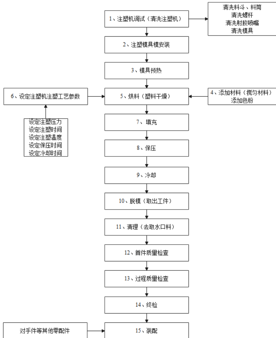
核心零部件生产工艺流程图
