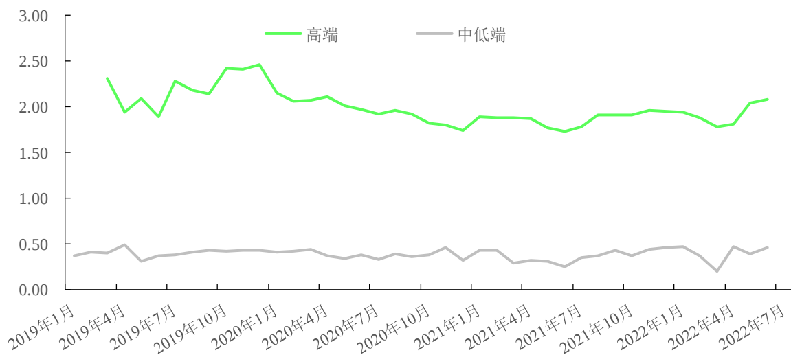
报告期内公司采购英飞凌 MEMS 芯片月度价格变动情况（单位：元/颗）
