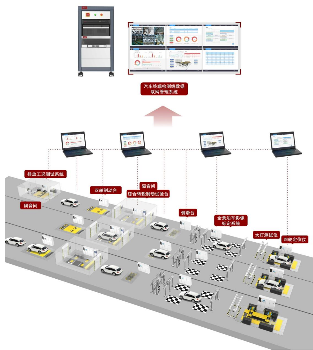
现代燃油汽车检测线布局示意图
