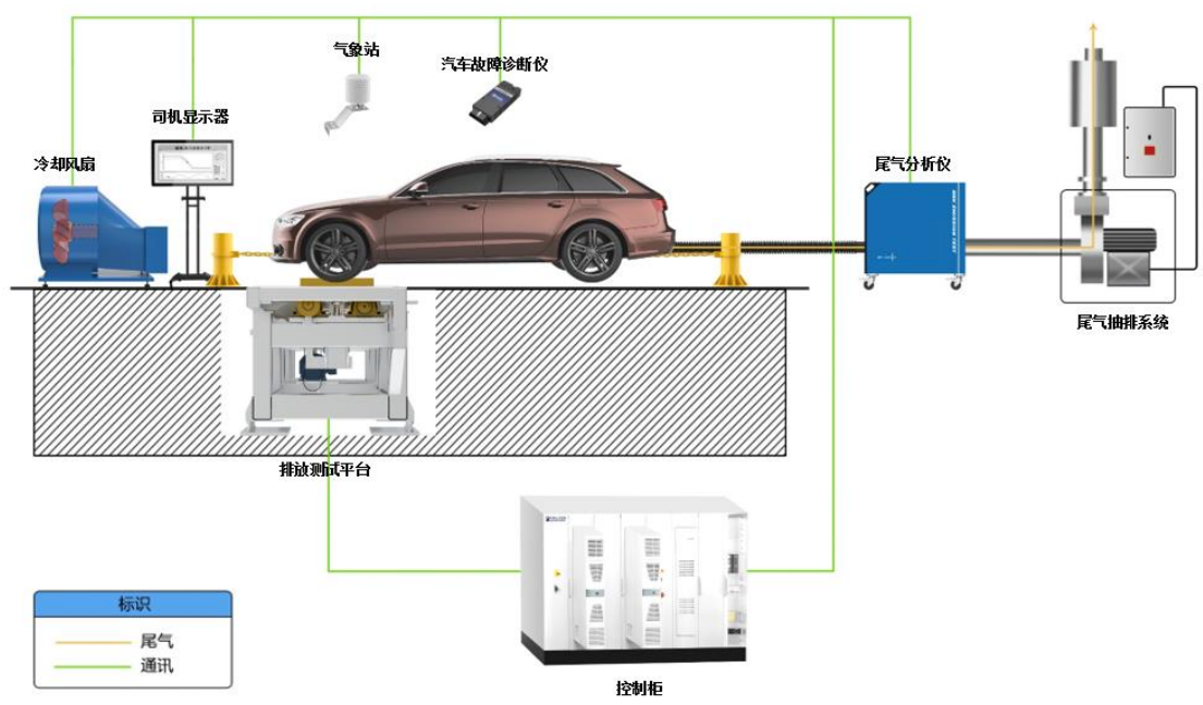
排放工况测试系统设计图
