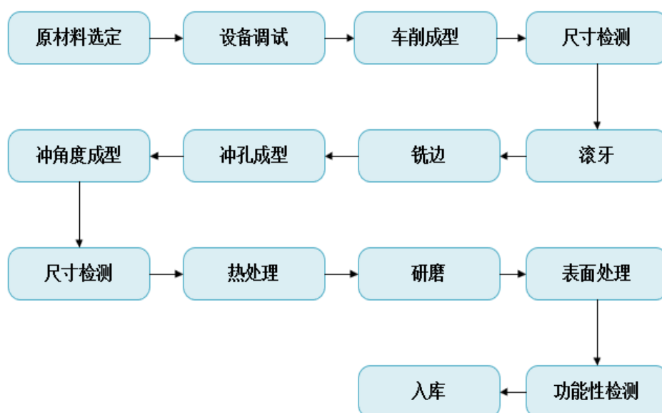
③CNC 件生产工艺流程图
