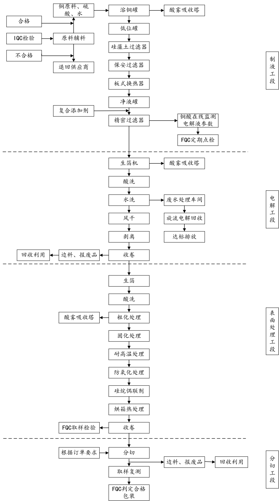
(1) 电子电路铜箔生产工艺流程图
