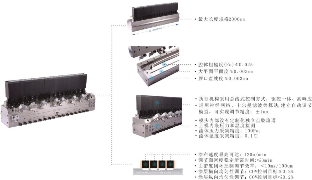
安全类智能款涂布模头
