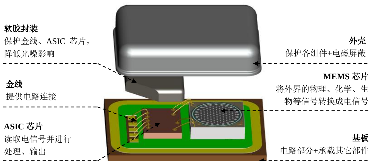
MEMS 声学传感器典型产品构造示意图
